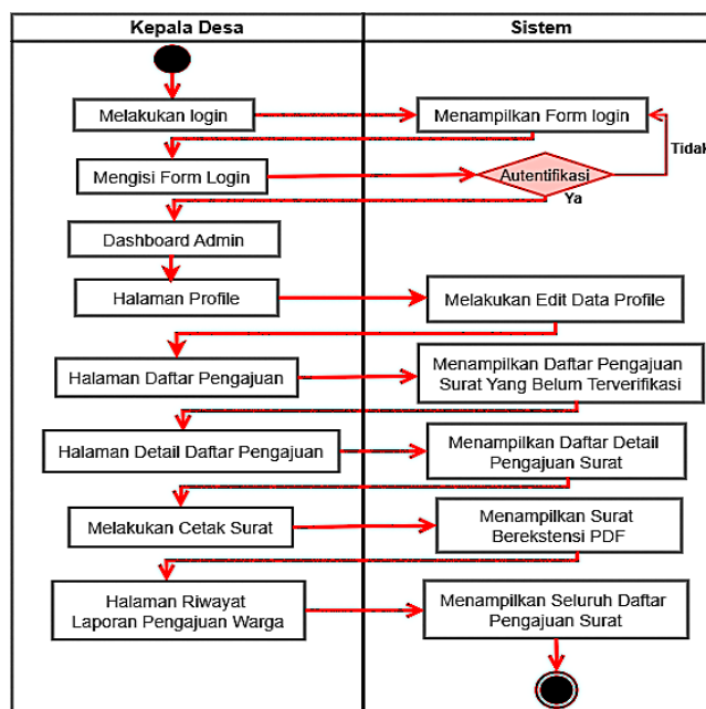
Gambar 7. Alur Proses Pengguna Kepala Desa
