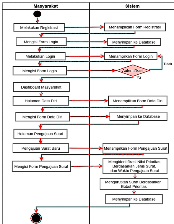
Gambar 5. Alur Proses Pengguna Masyarakat
