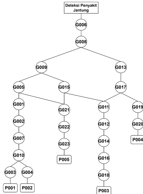
Gambar 6. Pohon Keputusan
